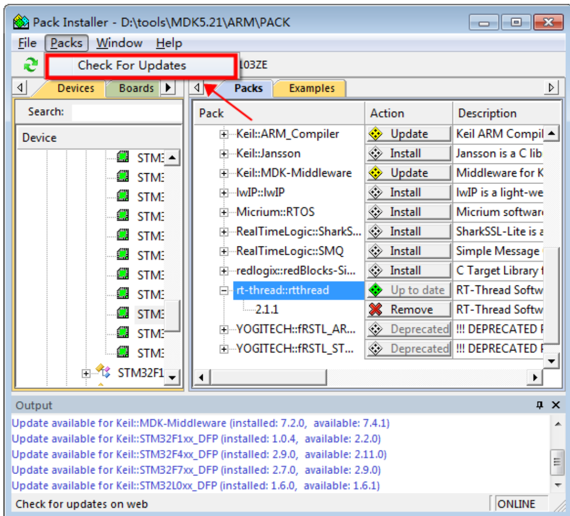
图 3: Pack Update
