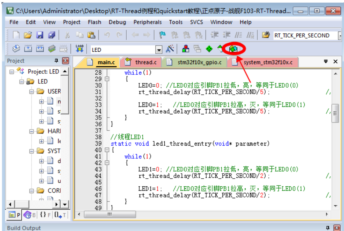
图 1: MDK5 主界面
